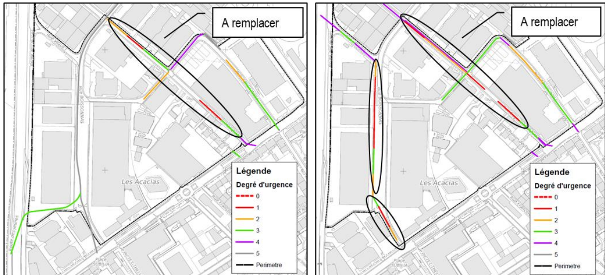
Figure 5 : Etat des collecteurs EU / EM, à gauche, et EP / EM, à droite.
