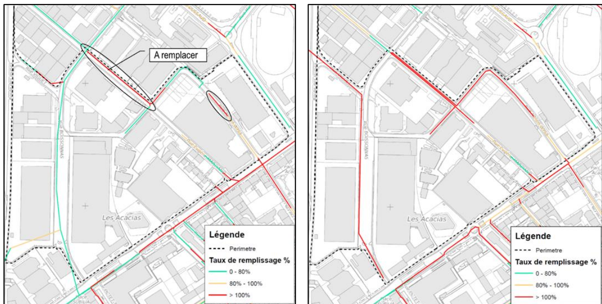
Figure 6 : Taux de remplissage des collecteurs EU / EM, à gauche, et EP / EM, à droite.
