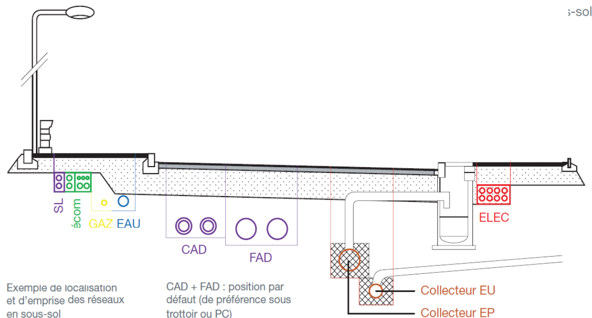
Figure 11 Exemple de localisation et d'emprise des réseaux en sous-sol issu du guide de conception et de coordination des travaux en sous-sol par SIG.
