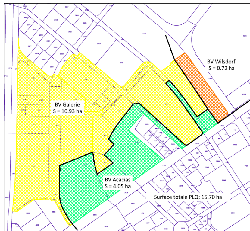
Figure 2 : Comparaison des bassins versants existants (PGEE) et projetés (PLQ).
