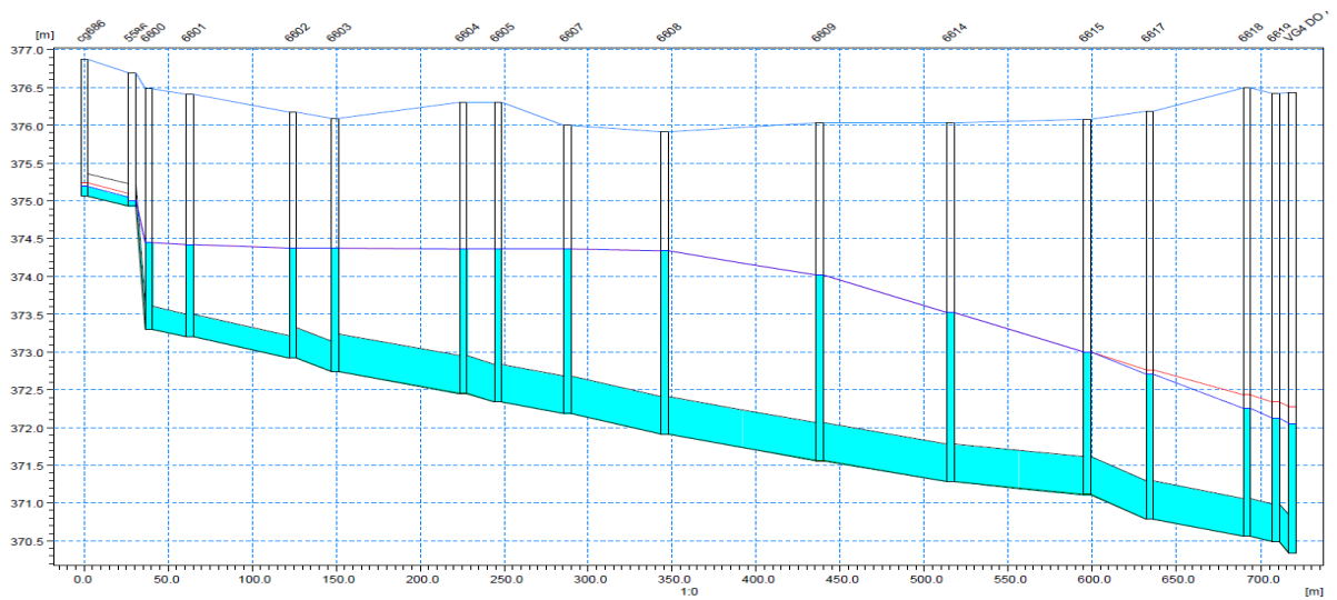
Figure 9 : Collecteur EU - Ligne d'eau T=10ans - Route Acacias selon PGEE.
