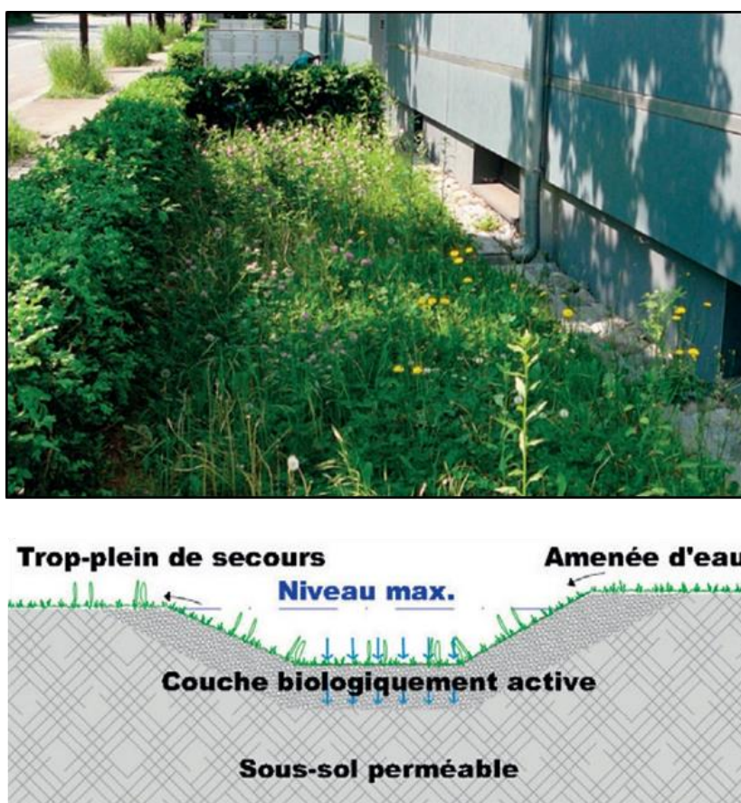
Figure 16 : Principe de rétention et d'infiltration (source VSA).
