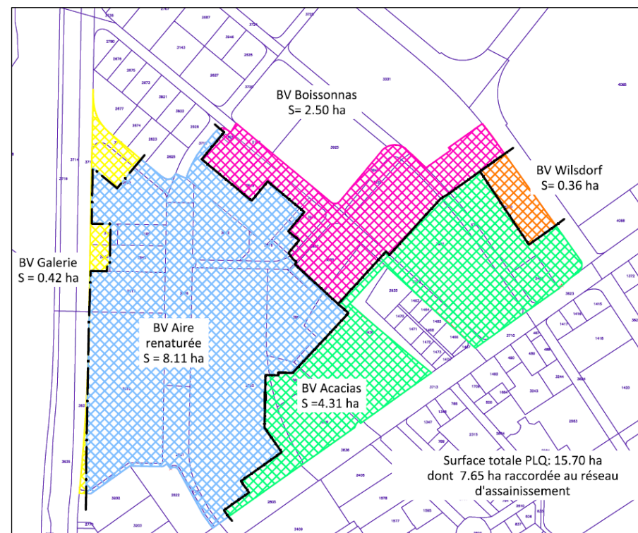
Figure 2 : Comparaison des bassins versants existants (PGEE) et projetés (PLQ).
