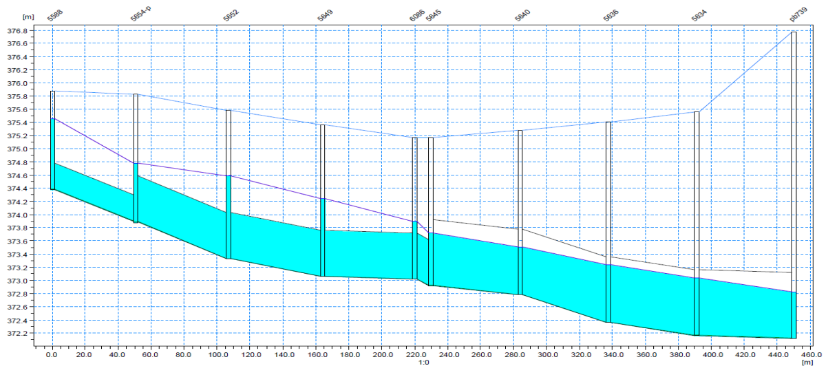
Figure 10 : Collecteur EP - Ligne d'eau T=10ans - Rue E. Marziano.
