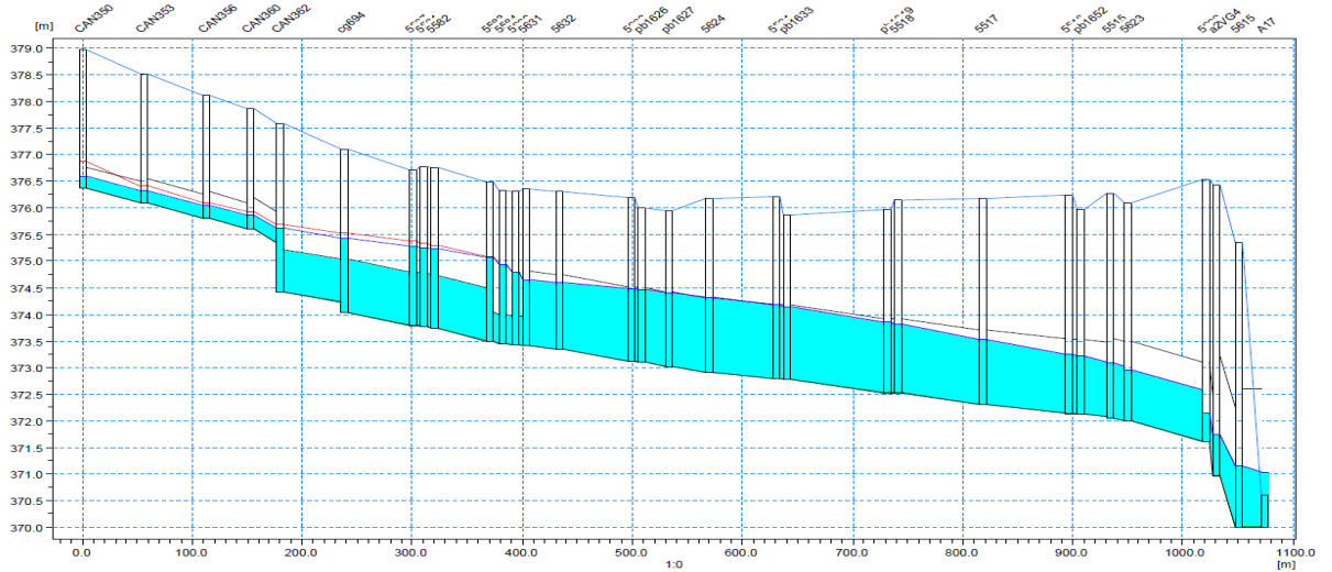
Figure 8 : Collecteur EP - Ligne d'eau T=10ans - Route Acacias selon PGEE.
