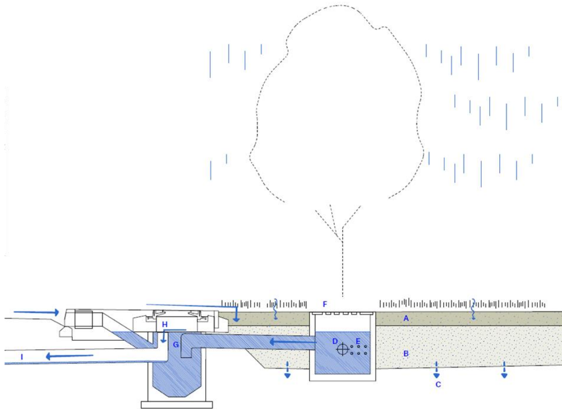
Figure 19 – Coupe de principe fosses de Stockholm – Système de diffusion et évacuation par trop plein des volumes excédentaires.
