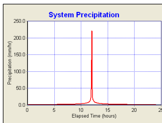
Figure 8 – Hyétochrome de pluie « IDF » pour T=10 ans et une durée de 24 heures.
