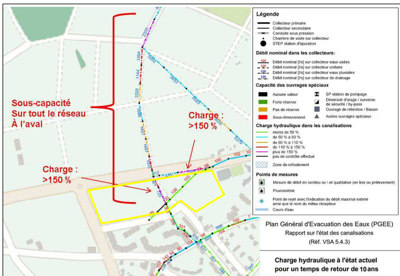
Figure 2 : Sous-capacité du réseau à l'état actuel, T=10 ans - PGEE
