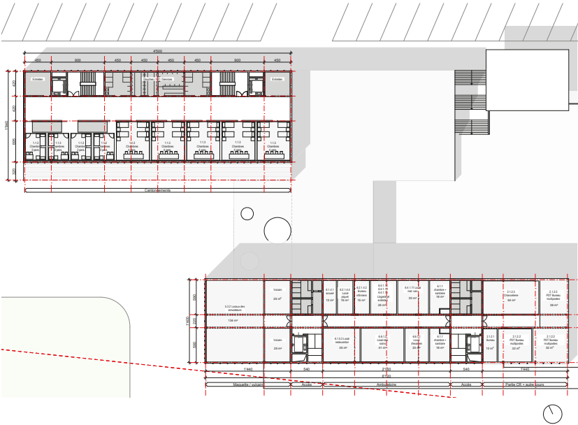
BATIMENT A, B ET C - NIV. +2
