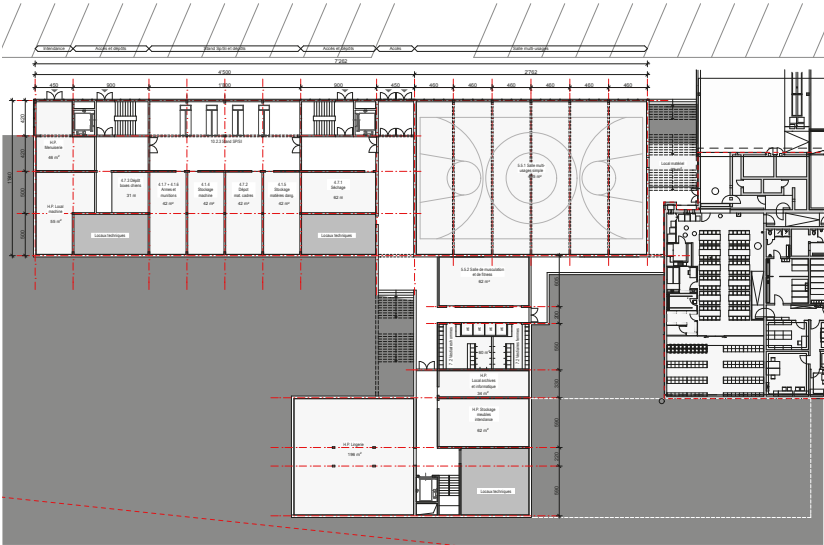
BATIMENT A, B ET C - REZ-DE-CHAUSSEE INFÉRIEUR - NIV. CHEMIN INTERNE ET STPA
