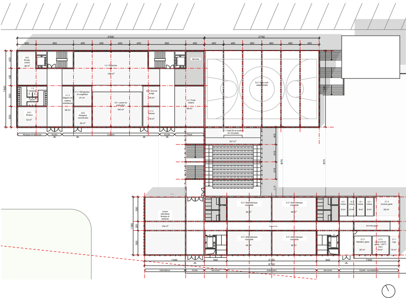
BATIMENT A, B ET C - REZ-DE-CHAUSSEE SUPERIEUR - NIV. ZONE VRTE ET TOITURE STPA
