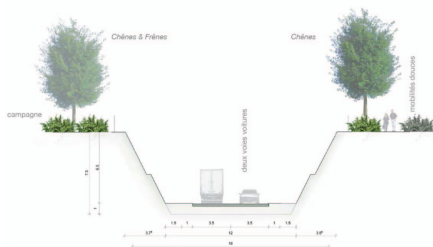
Profil en travers type et accompagnement paysager
