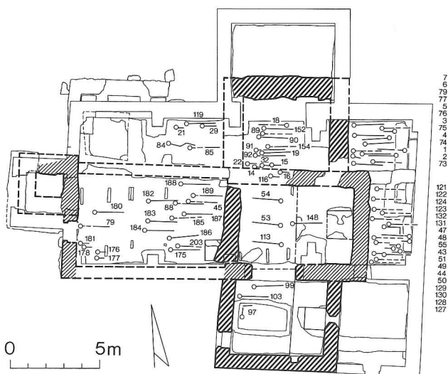
16. Plan de l'église à la fin du Moyen Age avec l'adjonction des chapelles Sainte-Catherine au nord et Notre-Dame au sud. L'autel du Saint-Esprit est posé contre le nouveau mur séparant le chœur de la nef, en avant des tombes 175 et 203. Les inhumations signalées sur ce plan correspondent aux sépultures aménagées entre le XIII e et le XVII e siècle (Dessin: J. Terrier).
