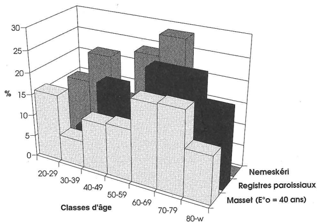
2. Eglise de Thônex, confrontation de la mortalité historique (registres paroissiaux) et de la mortalité estimée sur les squelettes (méthodes d'Acsádi et Nemeskéri, et de Masset).
