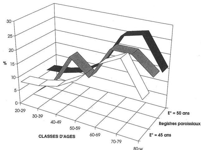
3. Eglise de Thônex, estimation de l'espérance de vie à la naissance. Les deux courbes de mortalité E^0 = 45 et 50 ans ont été construites à l'aide des tables-types de mortalité (Ledermann, 1969, réseau 100).
