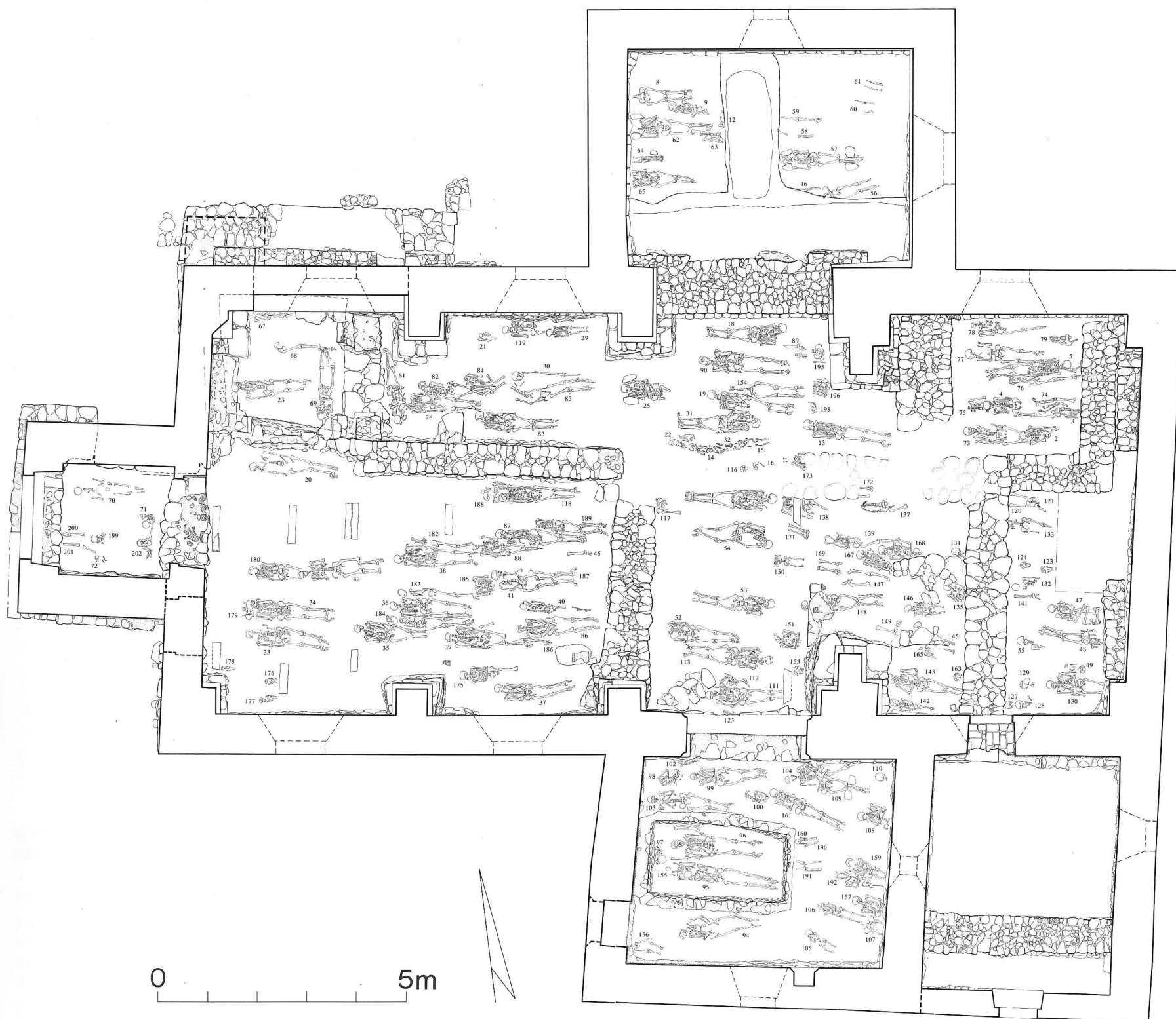
2. Plan général des fouilles (Dessin: J. Terrier).
