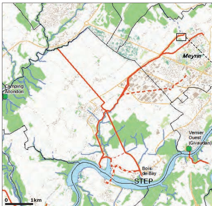
Réseau primaire des eaux usées (sitg, 2010)
